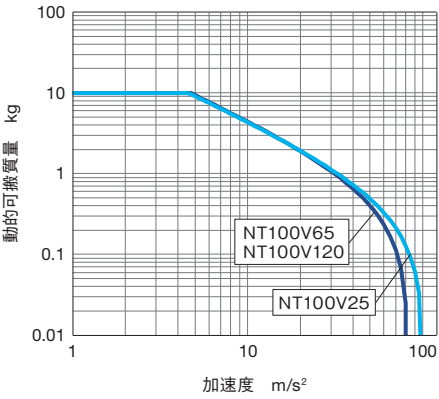
動的可搬質量
