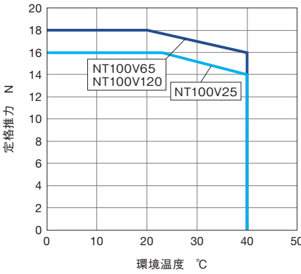
定格推力特性
