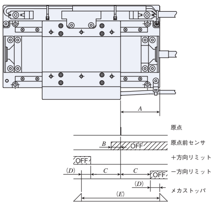
NT...V/RSCの場合(ケーブル引出し右方向)
