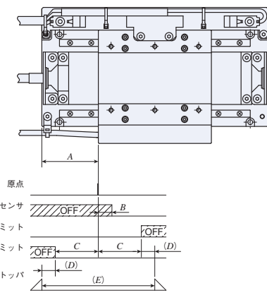
NT...V/LSCの場合(ケーブル引出し左方向)
