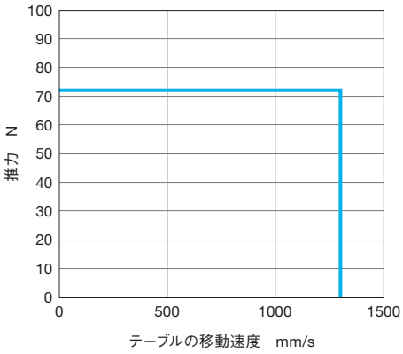
推力特性
